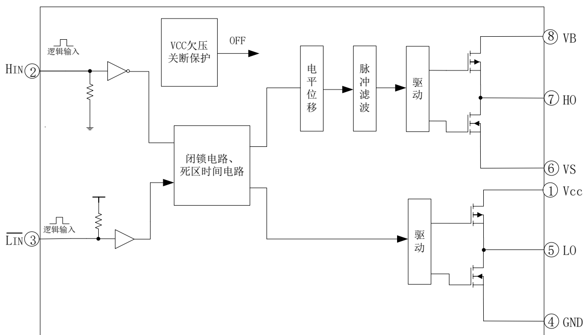
图 5-1. EG3023S 内部电路图
