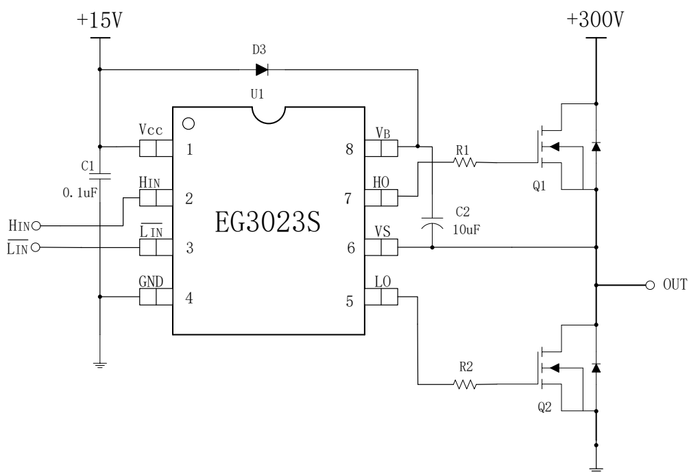
图 6-1. EG3023S 典型应用电路图
