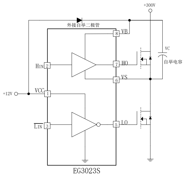
图 8-3. EG3023S 自举电路结构
