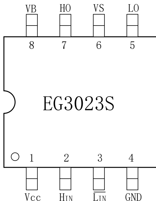
图 4-1. EG3023S 管脚定义
